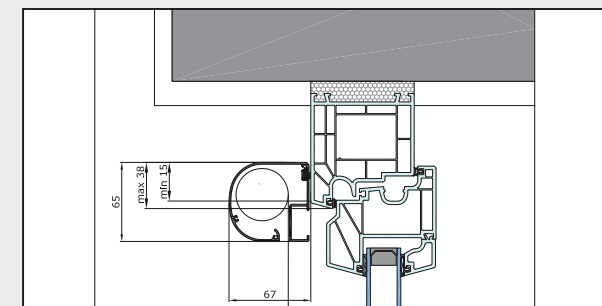
Platzbedarf oben
