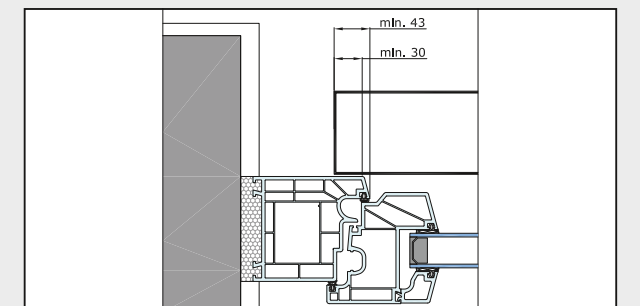
Platzbedarf seitlich
